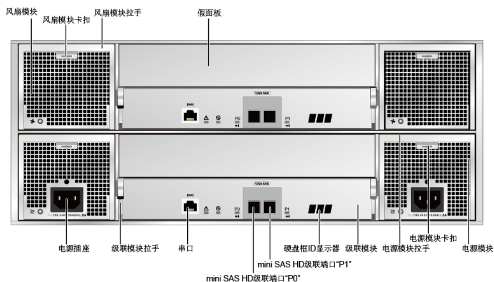
图1-64 硬盘框后视图
