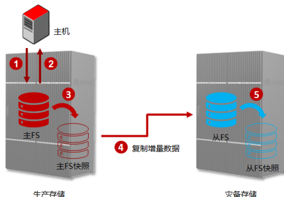
图1-97 文件系统异步远程复制原理
