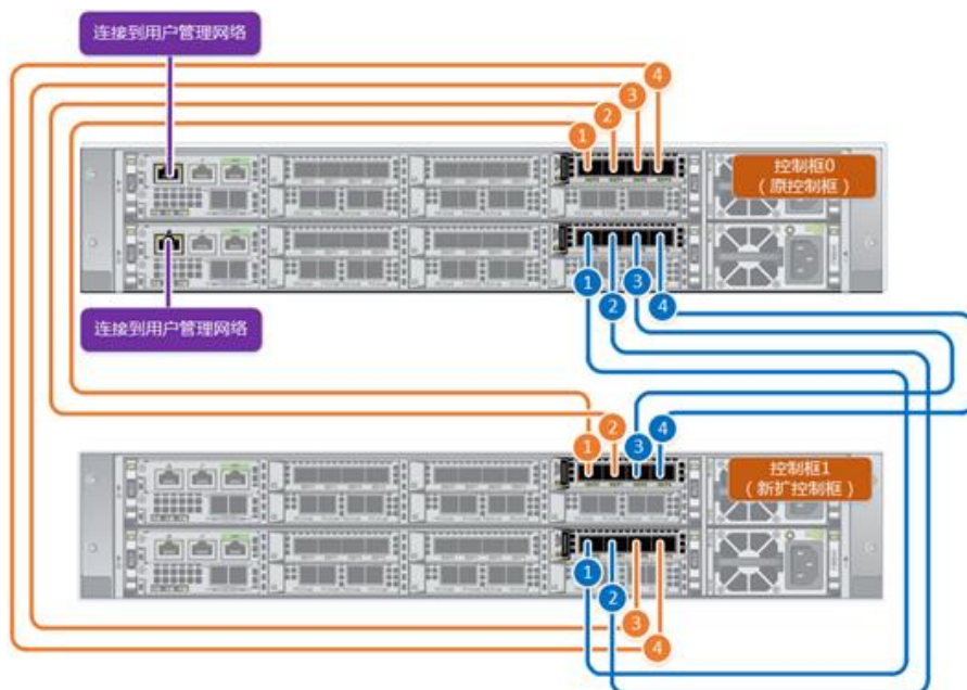
图1-75 图示：RDMA ScaleOut 4 控直连组网
