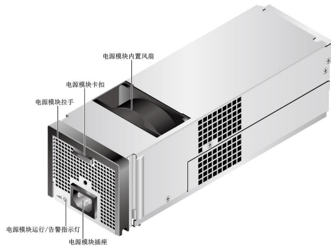
图1-69 交流电源模块
