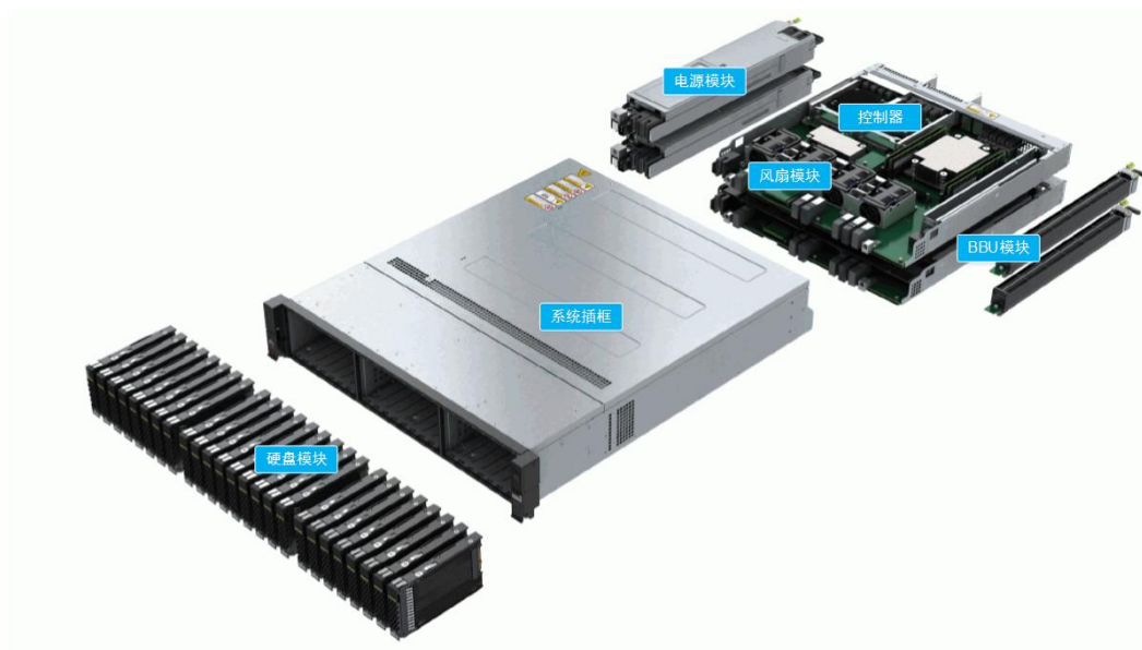
图1-16 2U 25 盘位控制框整体结构
