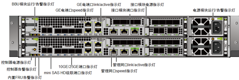
图1-28 控制框后面板指示灯
