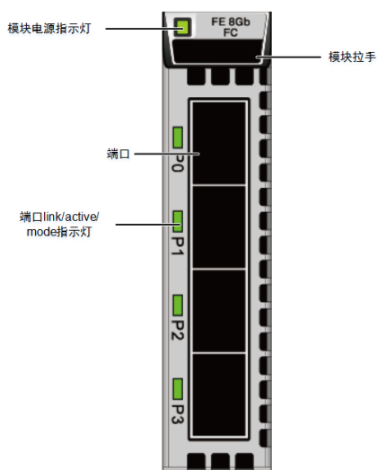
图1-51 速率为 8Gbit/s 的 TFCQ IO 接口模块
