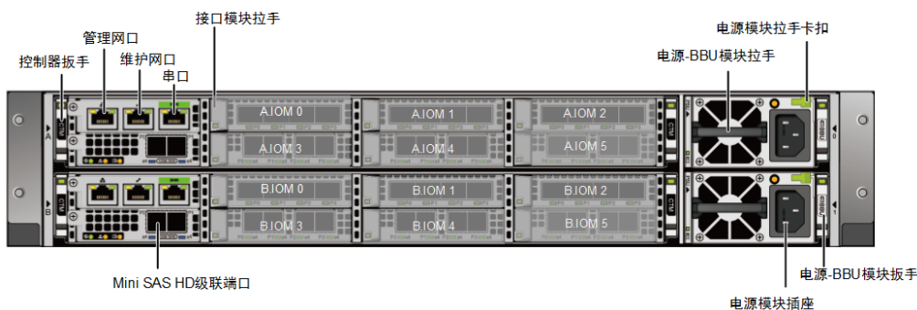
图1-34 控制框后视图（板载 100Gb RDMA 端口）
