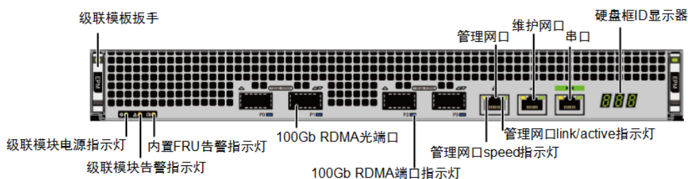
图1-71 级联模块接口信息
