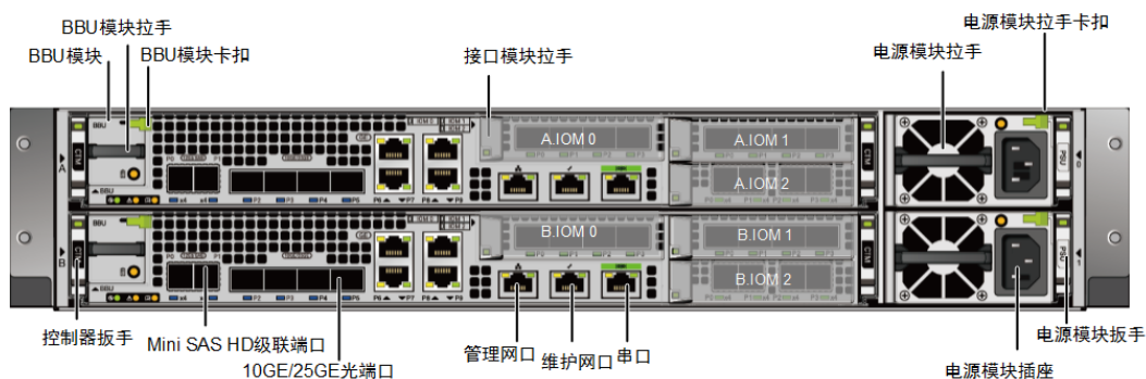
图1-18 控制框后视图
