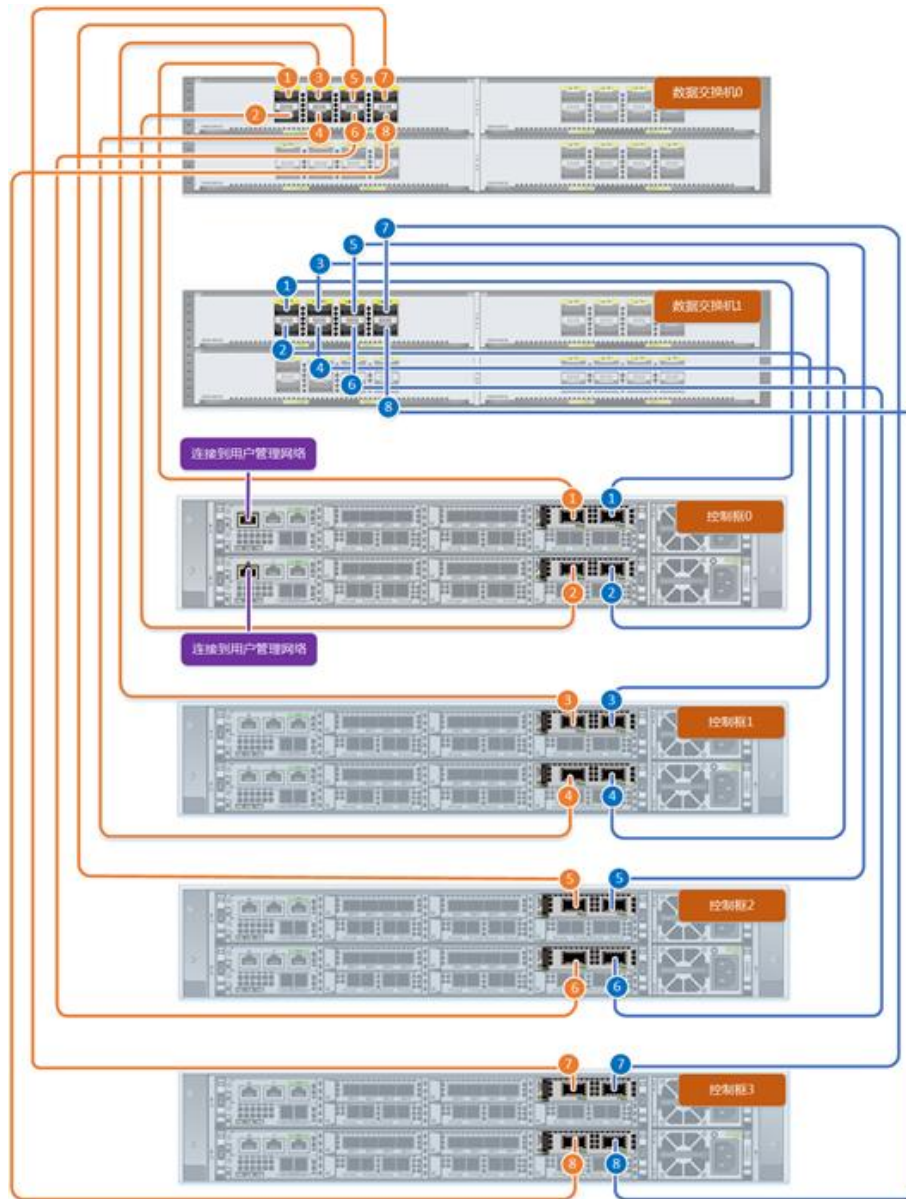
图1-76 图示：RDMA ScaleOut 8 控交换组网
