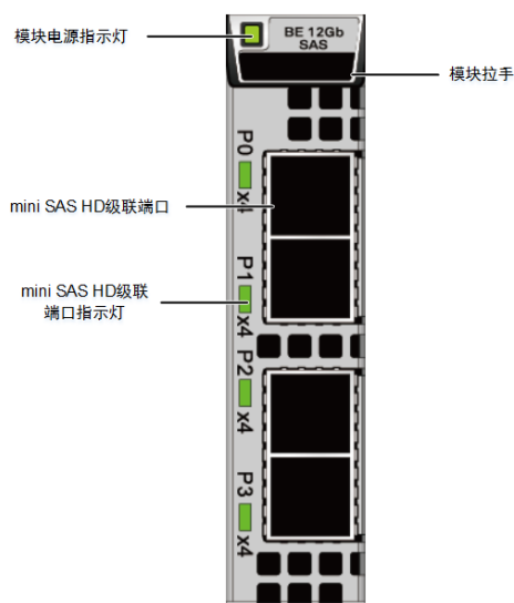
图1-56 12Gb SAS 级联模块
