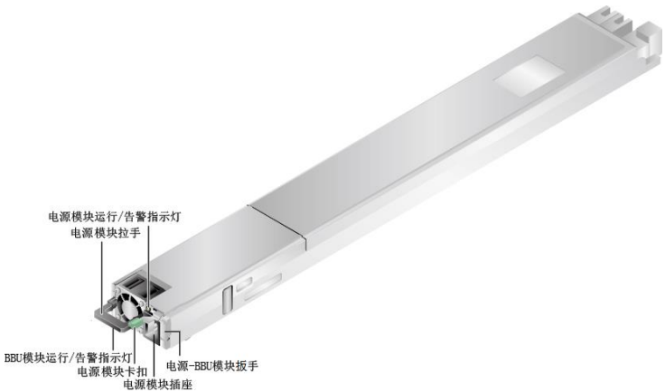
图1-40 电源-BBU 模块后视图
