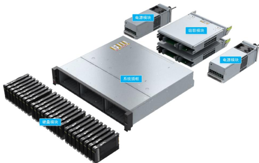
图1-58 2U 硬盘框整体结构
