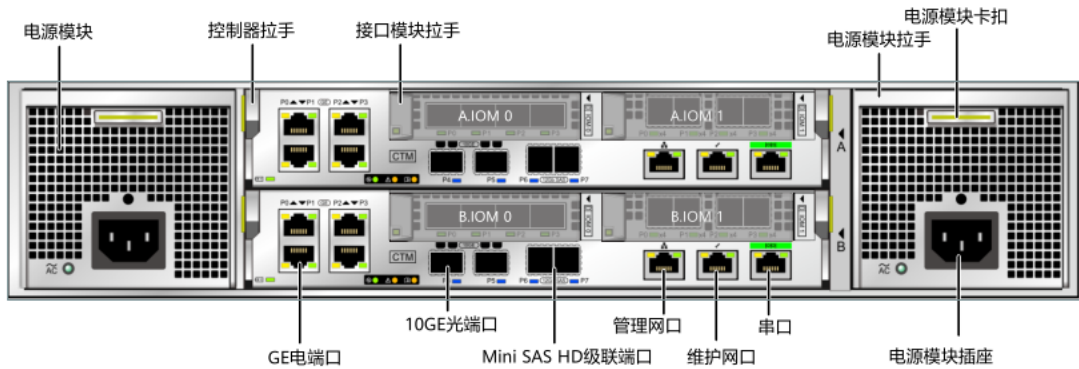
图1-15 控制框后面板指示灯
