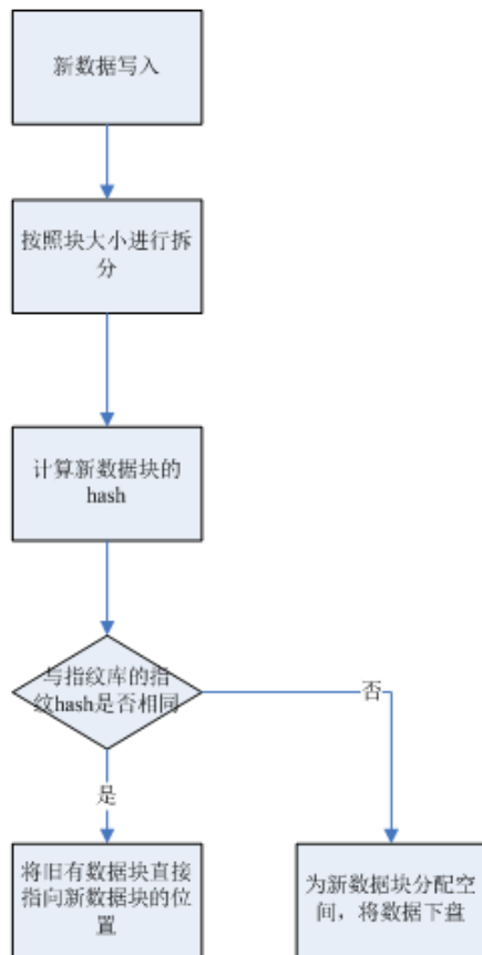
图1-81 重复数据删除处理流程
