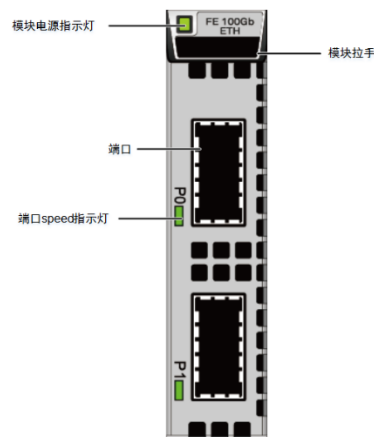
图1-48 100GE 接口模块
