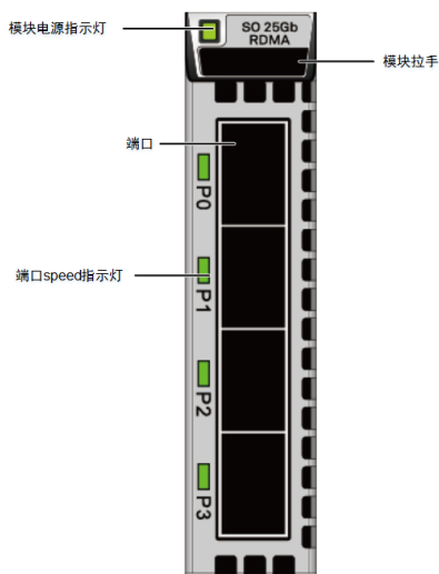
图1-46 25Gb RDMA 接口模块
