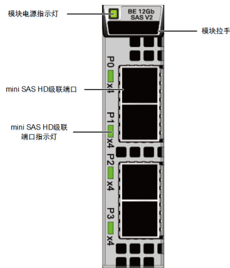
图1-57 12Gb SAS V2 共享级联模块
