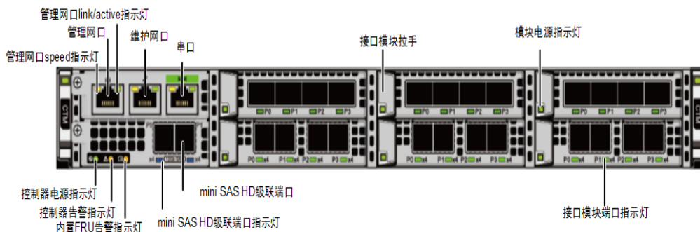
图1-37 控制器接口信息
