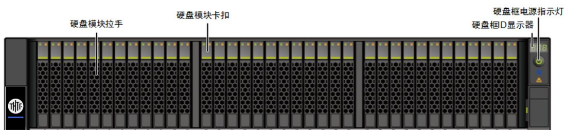
图1-62 硬盘框前视图
