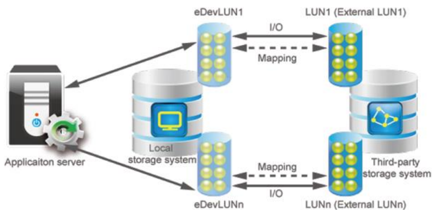
图1-80 异构虚拟化技术示意图
