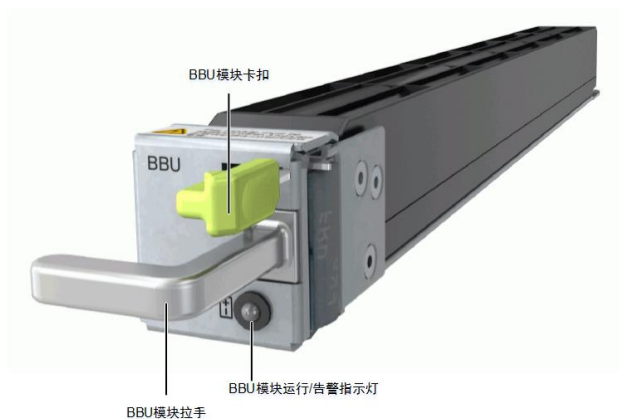
图1-23 BBU 模块前视图
