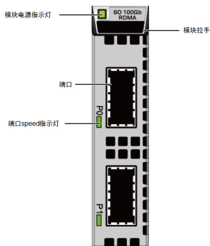
图1-49 SO 100Gb RDMA 接口模块
