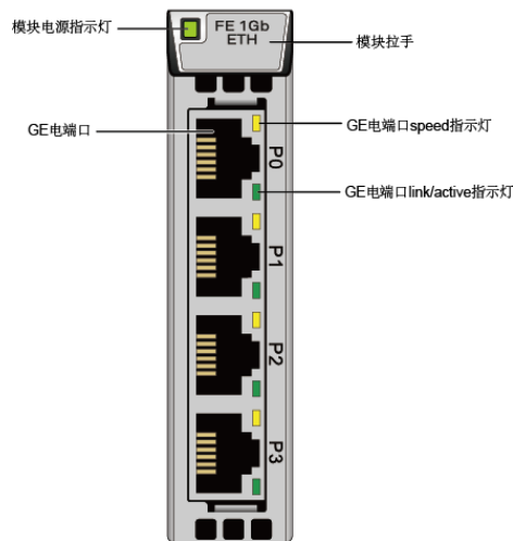
图1-45 GE 电接口模块
