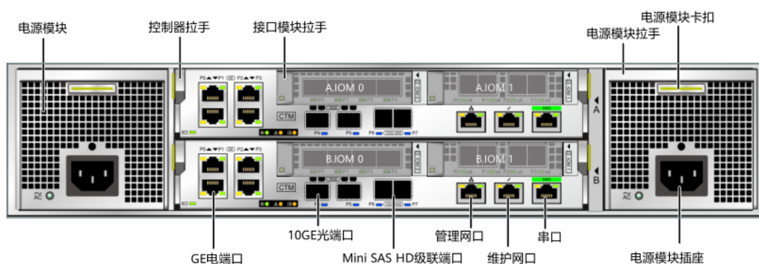
图1-7 控制框后视图
