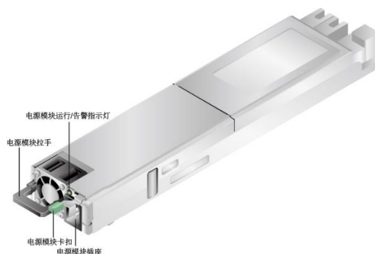
图1-73 交流电源模块
