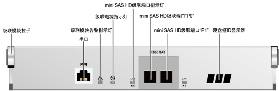
图1-68 级联模块接口信息
