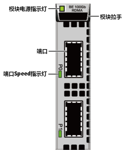
图1-50 BE 100Gb RDMA 接口模块
