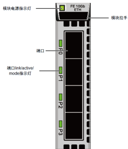
图1-52 速率为 10Gbit/s 的 TFCQ IO 接口模块
