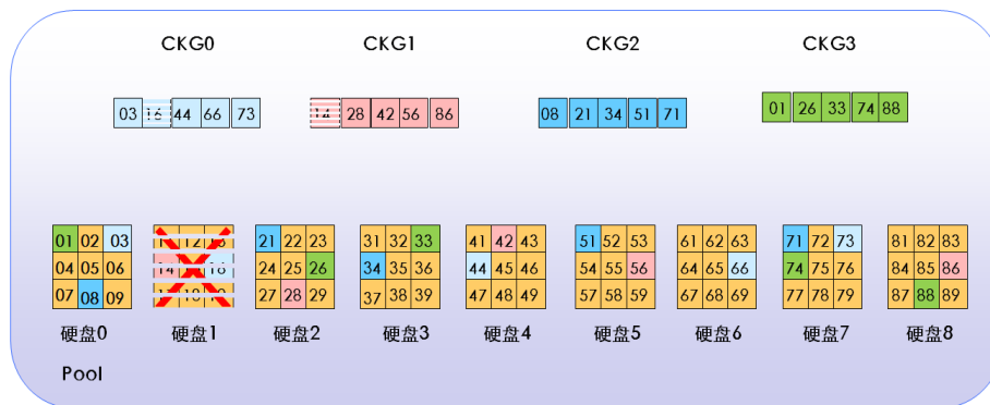
图1-78 RAID2.0+快速重构示意图（一）
