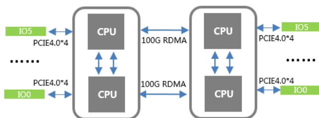
图1-74 高速总线背板互联
