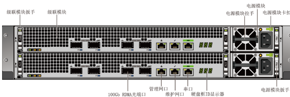
图1-65 配置交流电源模块硬盘框后视图
