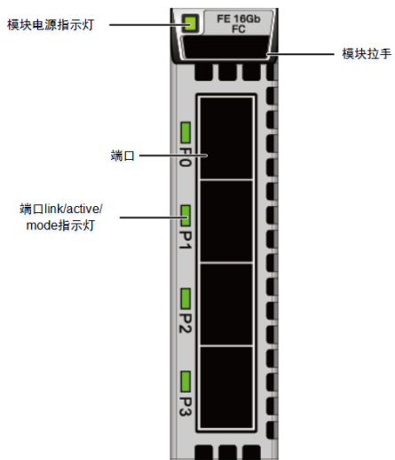
图1-53 速率为 16Gbit/s 的 TFCQ IO 接口模块
