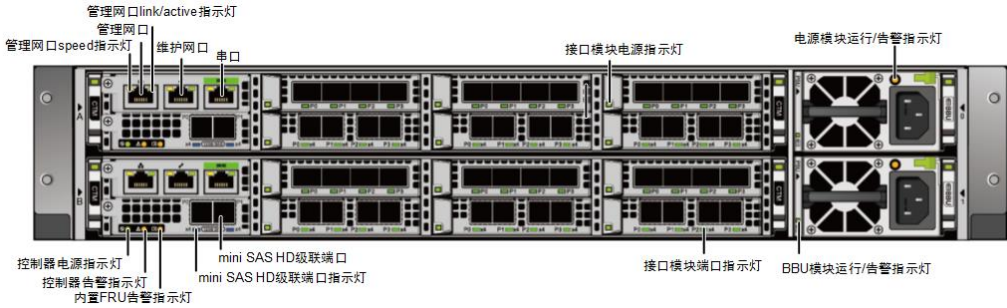
图1-44 控制框后面板指示灯
