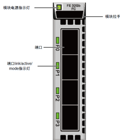
图1-55 速率为 32Gbit/s 的 TFCQ IO 接口模块
