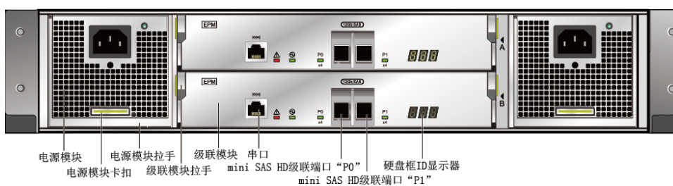
图1-63 硬盘框后视图
