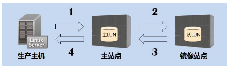
图1-93 同步复制技术原理示意图
